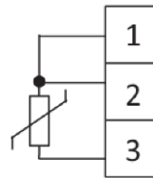
3-fils 2)
