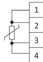
4-fils 2)
